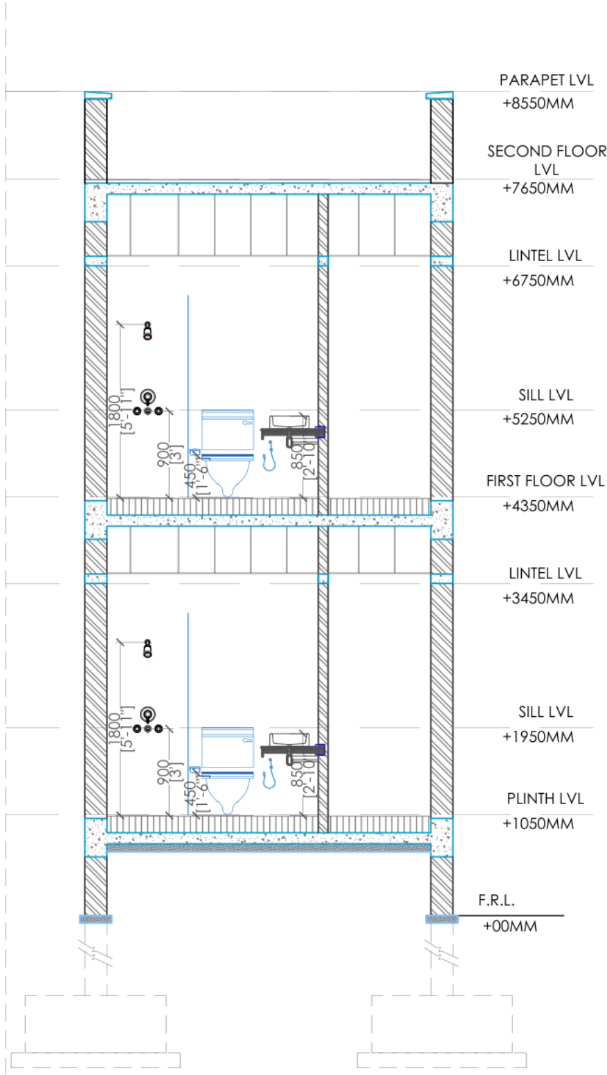
SECTION D-D
