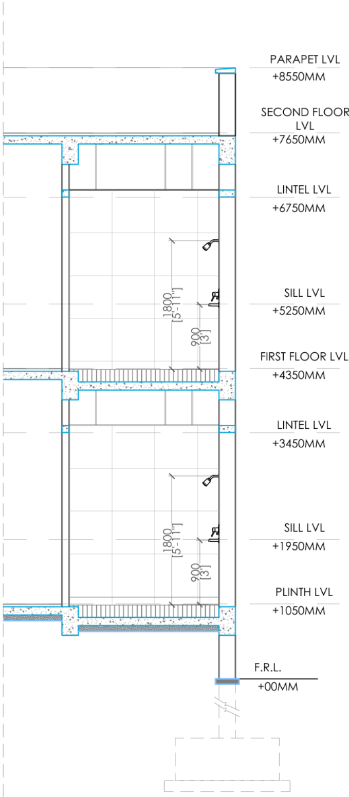
SECTION A-A
