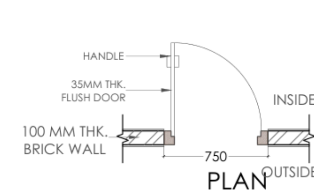
D3 - 750 x 2100 MM
